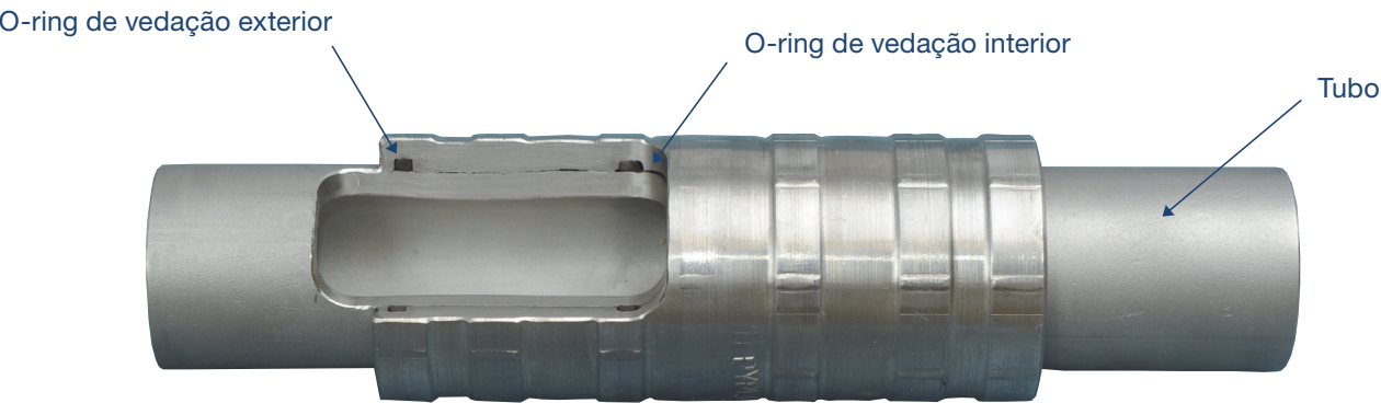
As conexões Pyplok® podem ser utilizadas em tubos de aço inox, duplex, super duplex, aço carbono e cobre-níquel.
