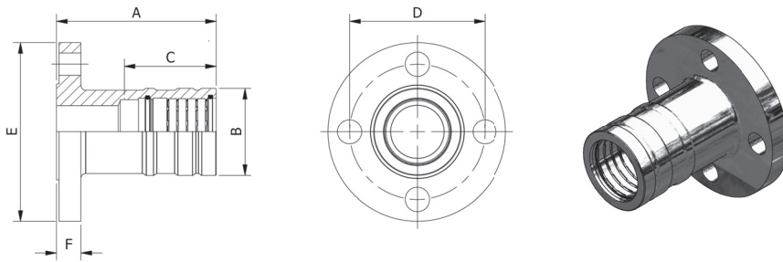
Flange - ANSI 300#, NPS - DM20019
