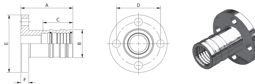
Flange – ANSI 600#, NPS - DM20027
