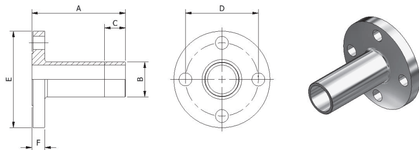
Flange - ANSI 300# x NPS Pipe - DM20119
