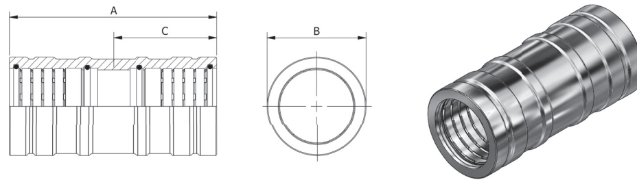
Coupling, OD Tube - DM60001
