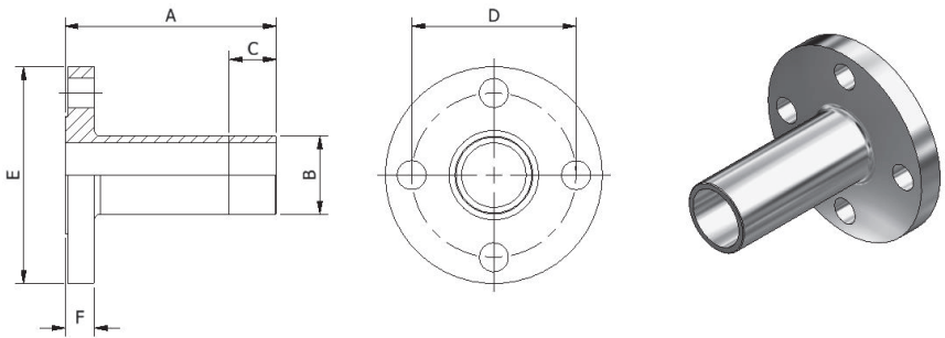
Flange - ANSI 150# x NPS Pipe - DM20118
